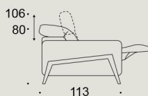
Poltrona 1BR
